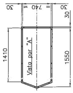
VISTA SUPERIOR TOLVA STANDARD PRENSA SIN DESATASCADOR
