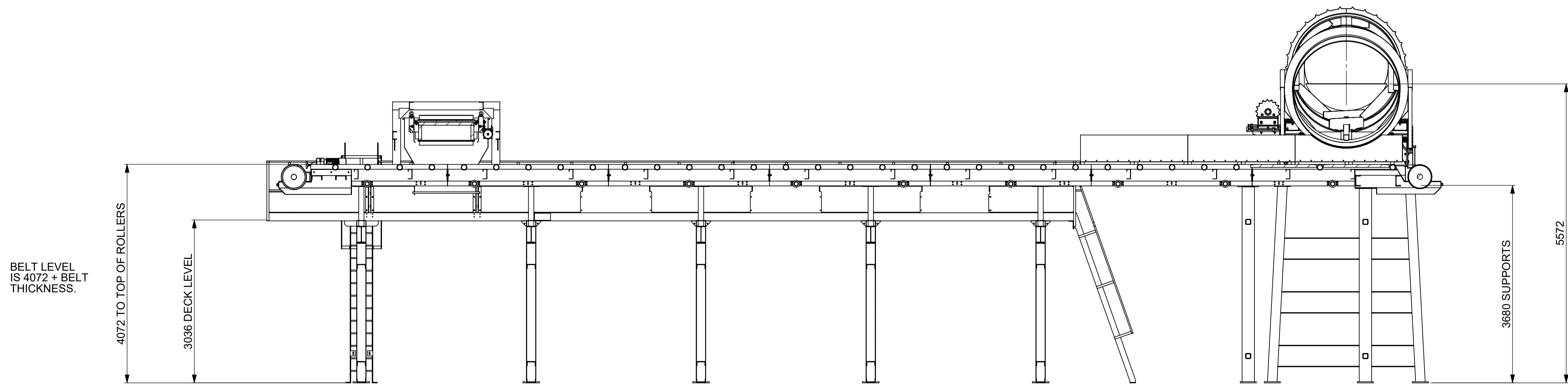
SECTION A-A
